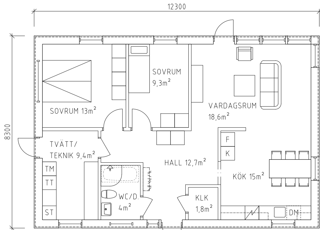
PLAN 1:100
